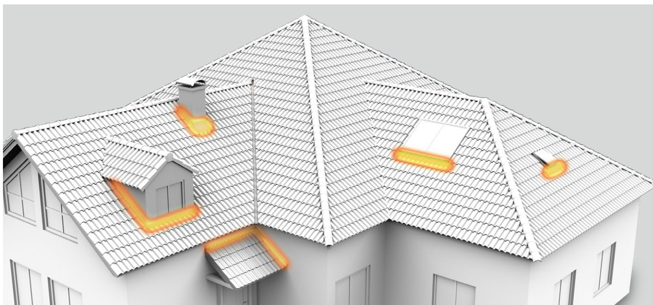
Wakaflex: tihenduslint seinte, korstnate ja teiste komponentide veetihedaks ühendamiseks katusega.
