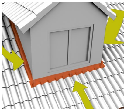
Vintskappide liidete tihendus.
